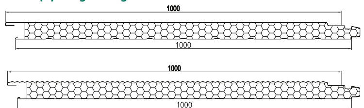
3d. Loại sóng nhỏ tăng cứng bên ngoài. BWE-1000BT
