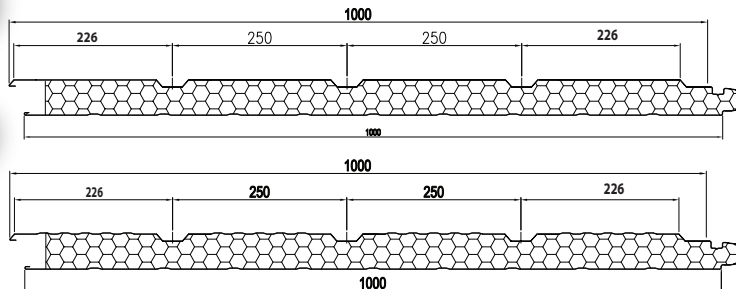
3f. Loại sóng nhỏ tăng cứng bên ngoài. BWE-250BT
